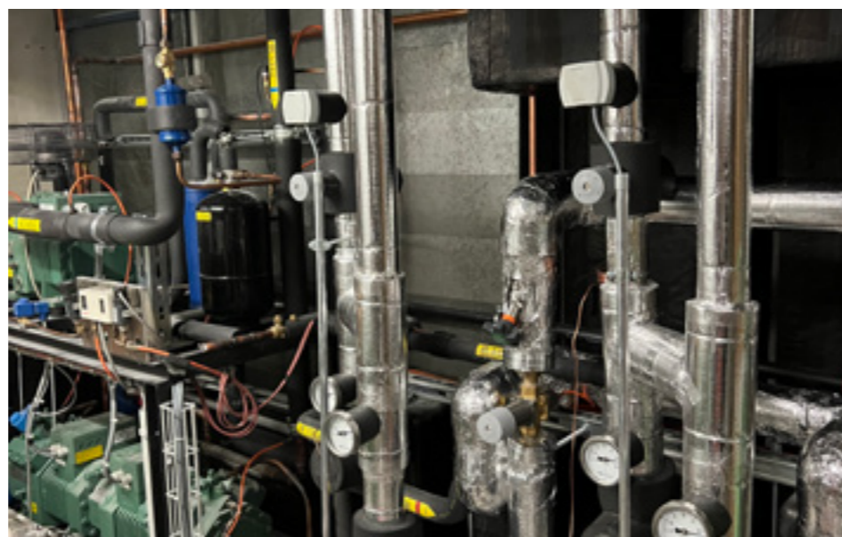
Wärmerückgewinnung von der Kältetechnik in den Wärmepumpenkreislauf
